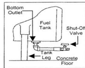
Bottom Outlet
